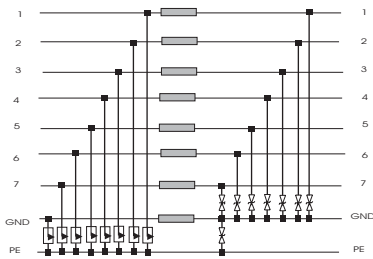
Fig2.- Conexión de un sistema punto a punto / Connection of system one to one.
